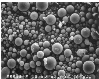
Afbeelding 13 Asdeeltjes 2000x vergroot, bekeken met een rasterelektronenmicroscoop
