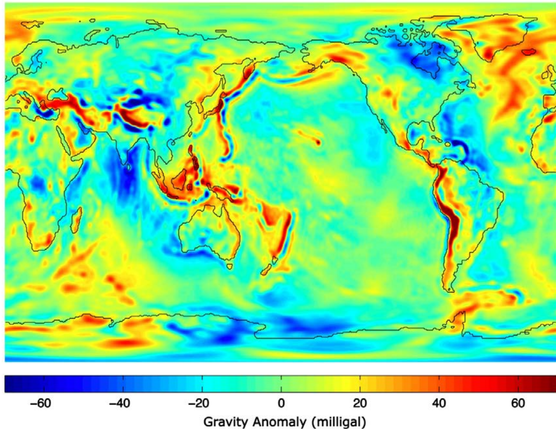
Afbeelding 41 Afwijking van de zwaartekrachtsversnelling, gemeten in \text{mGal} = 10^{-5} \text{ m/s}^2 .
