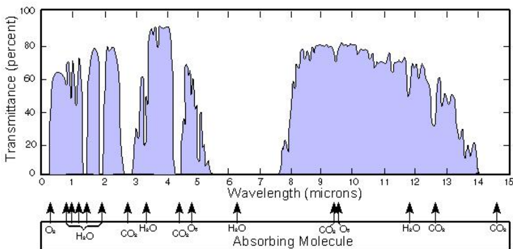
Afbeelding 24 Doorlaatbaarheid van de atmosfeer in het infrarood. Verschillende moleculen absorberen licht op verschillende golflengtes Bron: US Navy, via Wikimedia Commons
