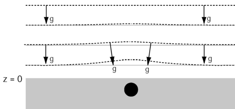
Afbeelding 37 Verschillende equipotentiaalvlakken en hun zwaartekrachtvector staan getekend voor een uniforme aarde met een lokale extra massa. De zwaartekrachtsvector staat altijd loodrecht op het equipotentiaalvlak. Bron: https://www.ualberta.ca/~unsworth/UA-classes/210/notes210/B/210B5-2008.pdf
