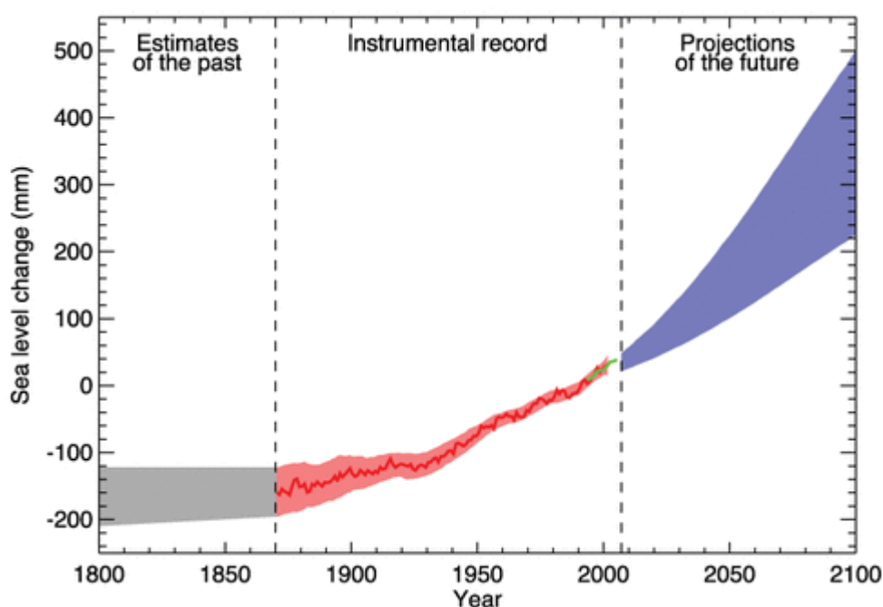
Afbeelding 46 Stijging van de zeespiegel in het verleden en voorspellingen voor de toekomst. De korte groene lijn is data verkregen via altimetrie Bron: IPCC Climate change science
