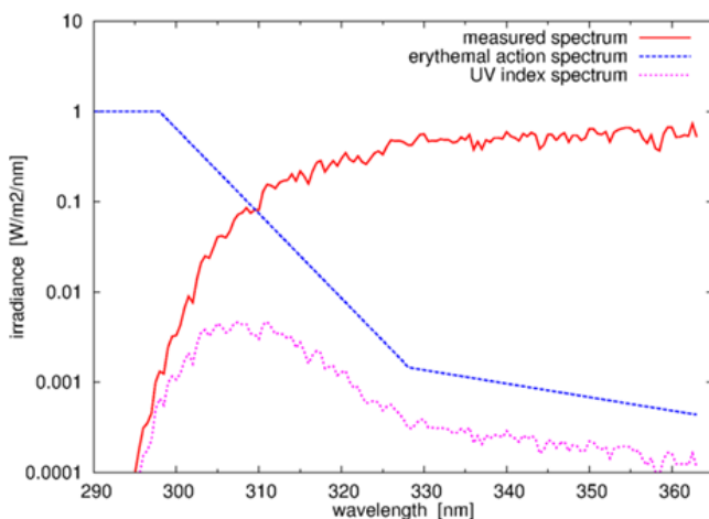
Afbeelding 50 UV index spectrum op basis van het erythema actiespectrum en een spectrum gemeten in De Bilt op 15 juni 2015. De UV-index is het oppervlak onder de curve van het UV-index spectrum. In dit voorbeeld is de UV index 6.202 (= 0.155 W/m².) Bron: KNMI
